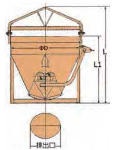
生コンバケツ (両開き)
