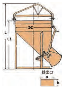
生コンバケツ (横出)
