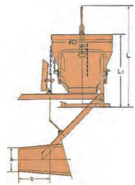
生コンバケツ (自在シュート)
