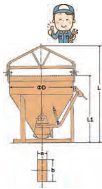
生コンバケツ (片開き)
