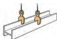
立吊クランプ ⚠ 安全上必ず2点吊り以上を厳守して下さい。
