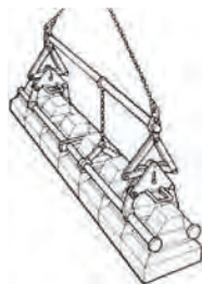
間知ブロック用クランプ
