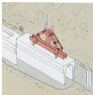
可変側溝吊クランプ
