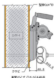
アイロンバイブレーター アイロン用分岐コード(5台接続可)
