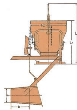
生コンバケツ (自在シュート)
