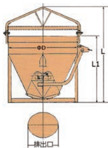
生コンバケツ (両開き)
