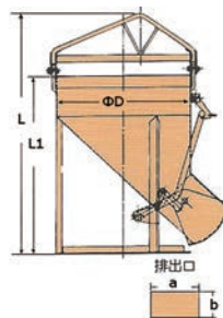
生コンバケツ (横出)
